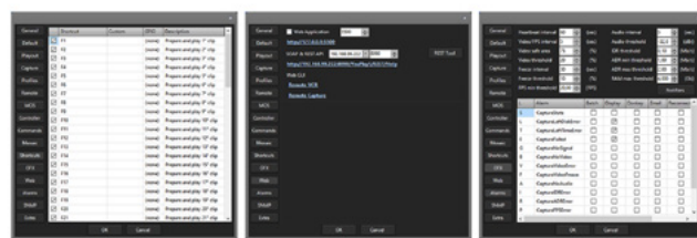
SHORTCUTS SETTINGS
